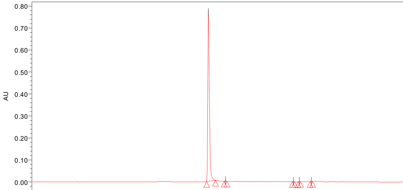
堆叠色谱图
